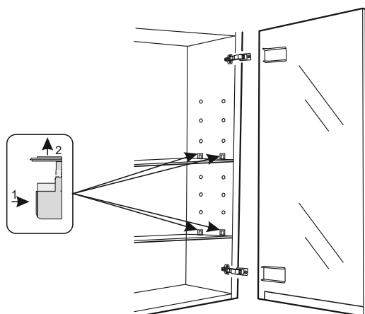
Montering demontering av glashyllor.
