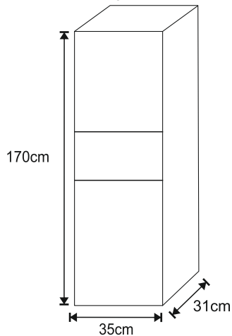
Sidoskåp 25
